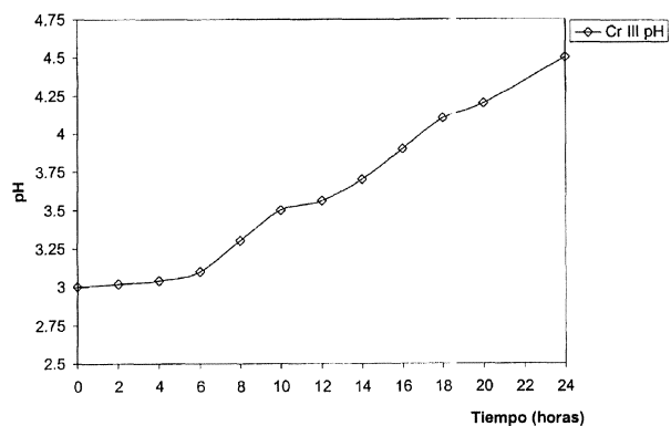
Figura 4. Comportamiento promedio del pH con respecto al tiempo, en el experimento realizado con Cr (VI).
