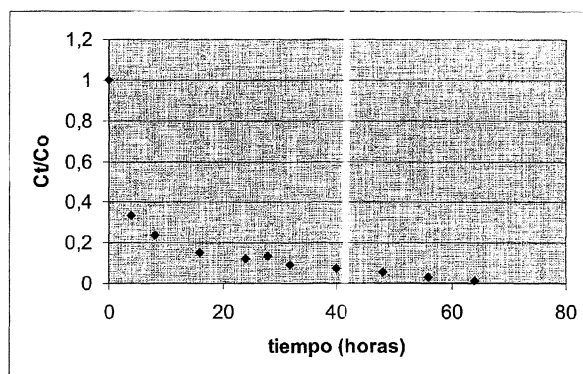
Figura 5. Concentración adimensional de Cr (III) frente al tiempo en condiciones de inmovilización del alga. Concentración inicial de Cr (III) de 85,6 mg/l a pH 4,5, biomasa algal soportada 200g/m 2 , área superficial del soporte 8,4 m 2 y volumen de trabajo 150 l.
