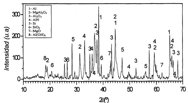
Figura 1. Diagrama de DRX del PAL inicial.
