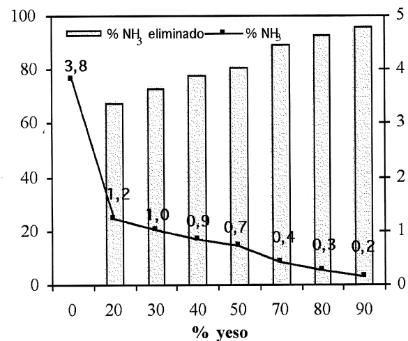
Figura 7. Evolución de la emisión de \text{NH}_3 junto con el porcentaje eliminado en las diferentes mezclas del PAL/yeso.
