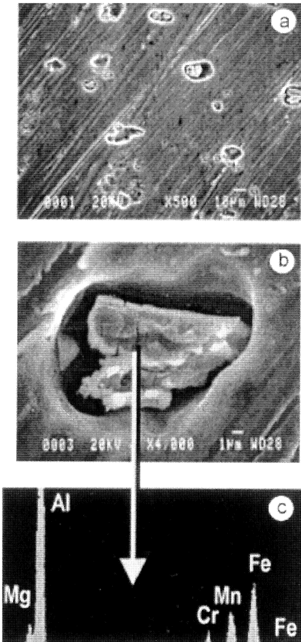
Figura 1. (a) Imagen S.E.M. de muestra tratada por inmersión en disolución aireada de NaCl al 3,5 % durante 6 h. (b) Detalle de zona corroída por alcalinización local. (c) Espectro E.D.S. sobre precipitado Al(Mn, Fe, Cr).
