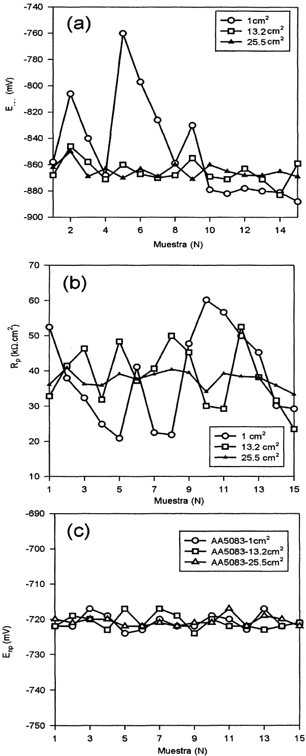
Figura 7. Parámetros electroquímicos obtenidos al exponer muestras con distinta superficie. (a) Potencial de corrosión (b) Resistencia de polarización. (c) Potencial de nucleación de picadura. Muestra: aleación AA5083. Medio: disolución de NaCl al 3,5 %.
