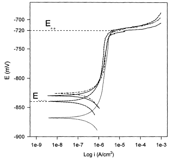
Figura 6. Curvas de polarización de muestras de la aleación AA5083 en disolución de NaCl al 3,5 %, durante las dos primeras horas. Superficie expuesta: 1 cm 2 .
