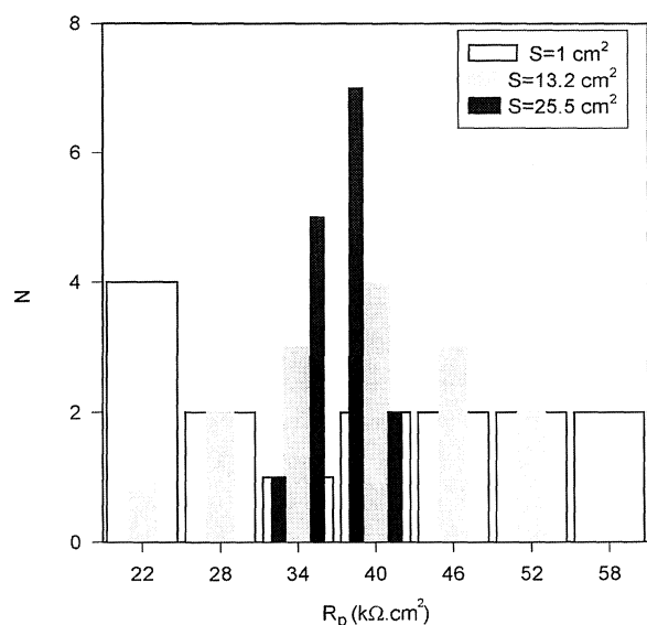
Figura 9. Distribución de frecuencias de la resistencia de polarización y del potencial de nucleación de picadura para las tres áreas estudiadas.
