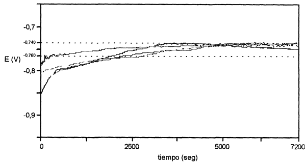
Figura 5. Curvas E_{corr} - t de muestras de la aleación AA5083 en disolución de NaCl al 3,5 %, durante las dos primeras horas. Superficie expuesta: 1 cm 2 .
