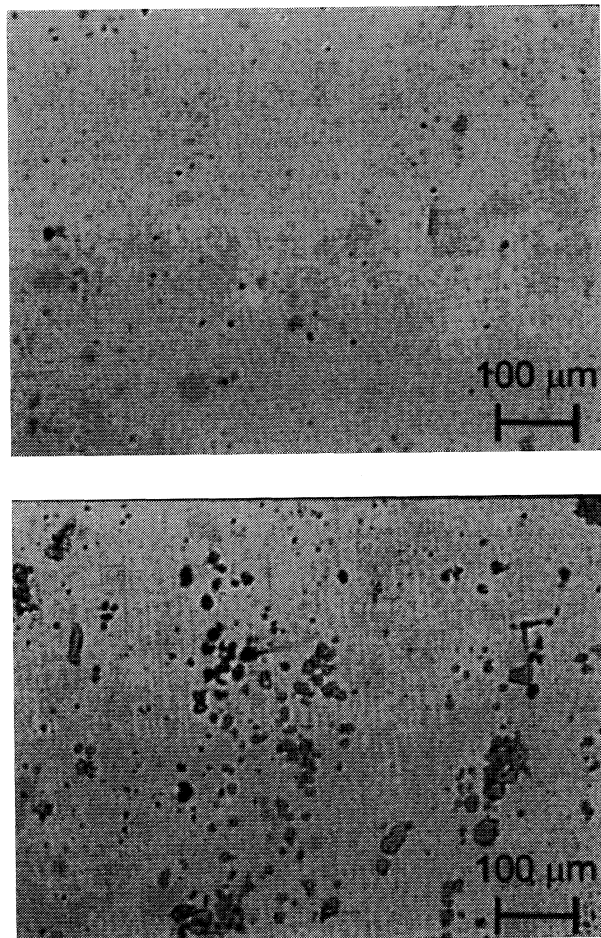
Figura 3. Imágenes de microscopía óptica de una muestra de la aleación AA5083 pulida hasta nivel especular. Zonas con distinta densidad superficial de precipitados.
