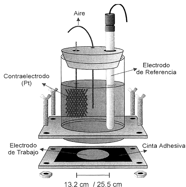
Figura 4. Celda de tres electrodos con superficie expuesta variable.
