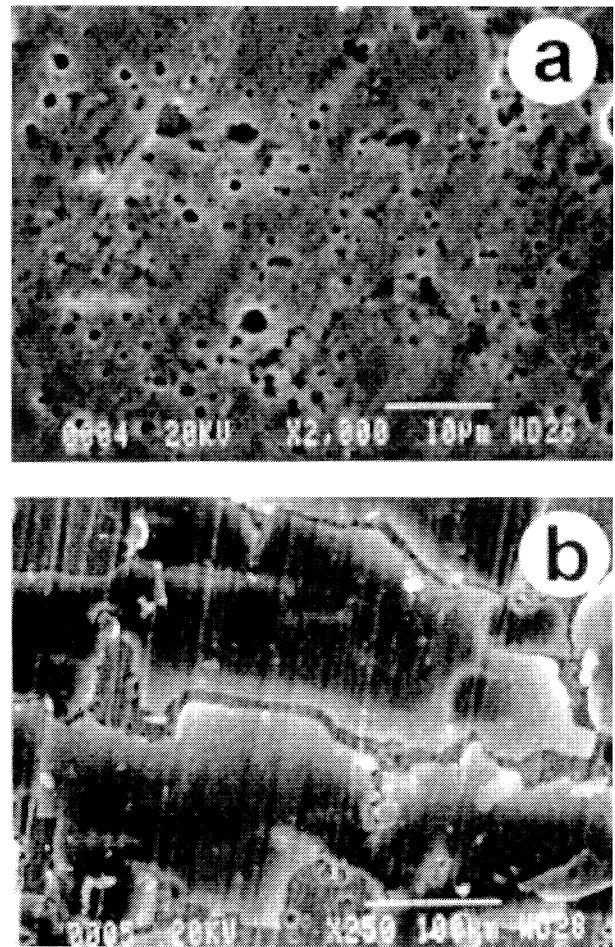
Figura 2. Imágenes S.E.M. de muestra de la aleación AA5083 tras 15 d de inmersión en disolución aireada de NaCl al 3,5 %. (a) Micropicaduras en muestra decapada. (b) Capa de óxido en muestra sin decapar.
