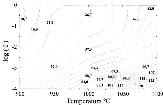
FIG. 6.— Isolíneas de tamaño de grano recristalizado en función de la temperatura y velocidad de deformación.
