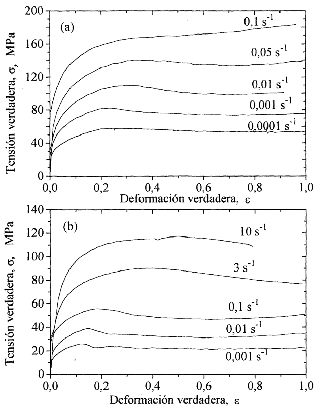
FIG. 1.— Curvas de fluencia del acero estudiado. a) 900 \text{ }^\circ\text{C} y b) 1.150 \text{ }^\circ\text{C} .
