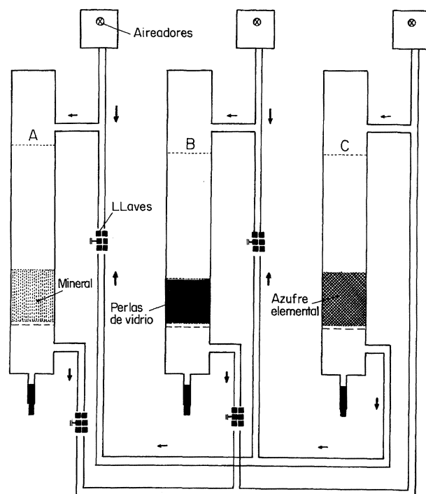
FIG. 1.— Esquema de instalación usado en la biolixiviación. Circuito 1: constituido por A y C. Circuito 2: constituido por B y C.
